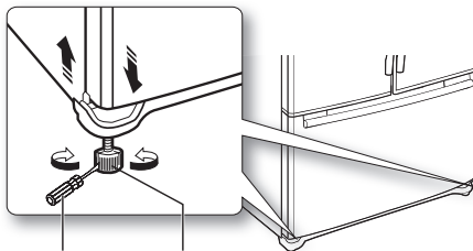
Ravan odvijač Podesiva nožica
