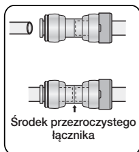
Łącznik typu A
