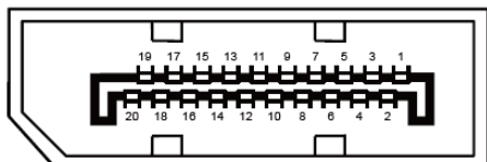
20-stykowy przewód sygnałowy kolorowego wyświetlacza
